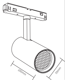
MG-20TS015
